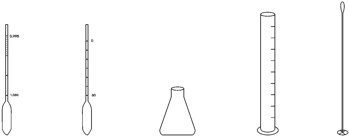
a) Tỷ trọng kế loại B b) Tỷ trọng kế loại A c) Bình tam giác d) Ống đo lường e) Que khuấy
